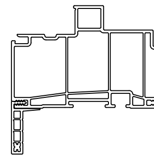
1" FLUSH FIN
