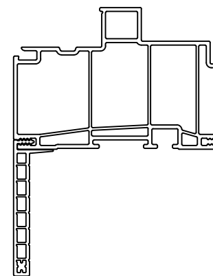
2" FLUSH FIN
